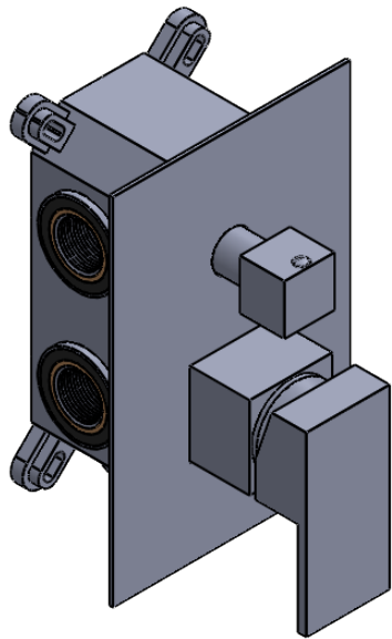
VISTA ISOMETRICA
