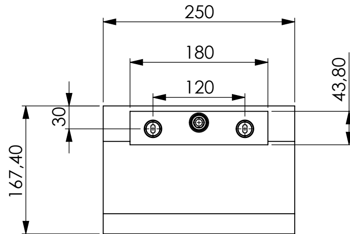
VISTA POSTERIORE
